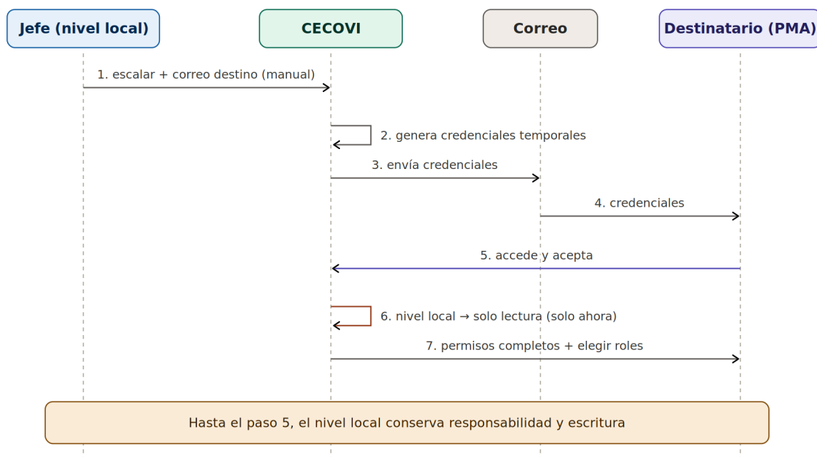
Figura 3. Secuencia de la transferencia con aceptación; la revocación solo ocurre tras aceptar.
