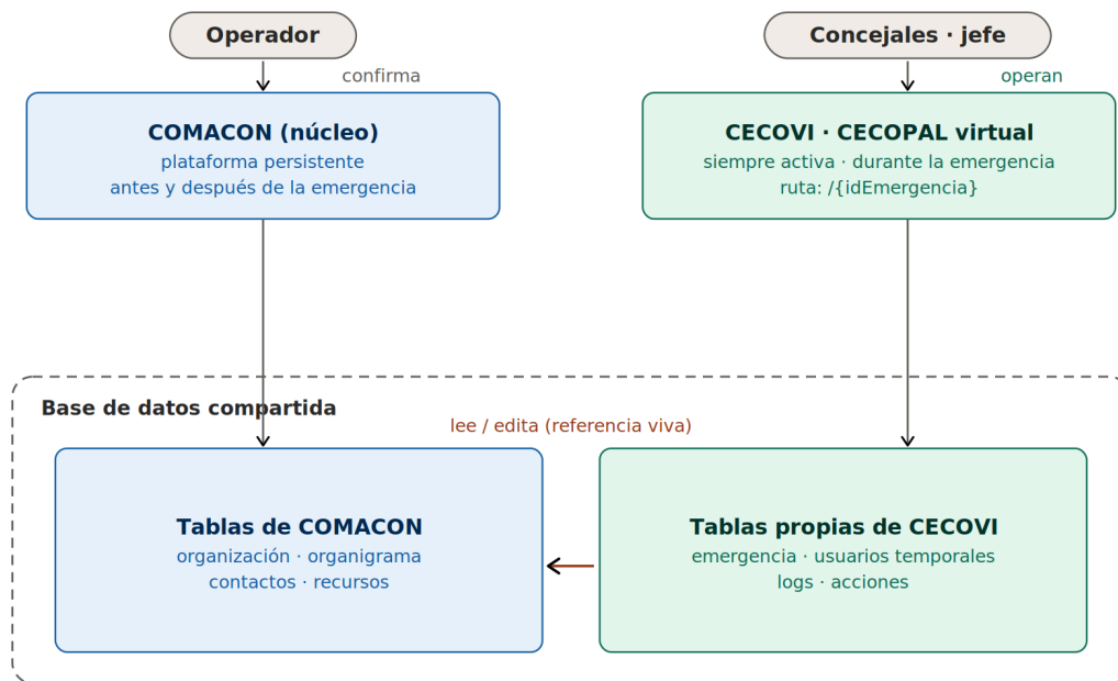
Figura 1. Contexto del sistema: las dos plataformas sobre una base de datos compartida.
