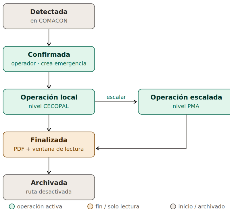
Figura 2. Ciclo de vida de la emergencia. El escalado es opcional y de un único salto.
